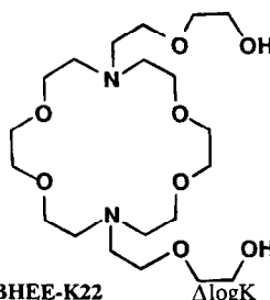
BHEE-K22
