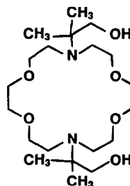
BDME-K22
