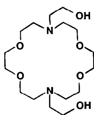
BHE-K22
